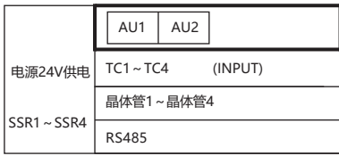
AC/DC 24V供电隔离框图
